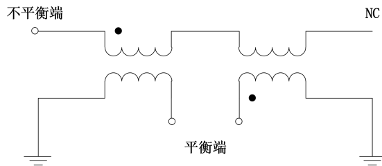
YLBL-19-E6-D产品原理图
